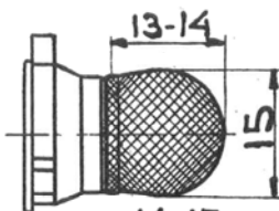
GLÖDNÄT GNAB-8 FÖR 8-LIT. BRÄNNARE.
