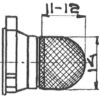
GLÖDNÄT GNAB-6 FÖR 6-LIT. BRÄNNARE.
