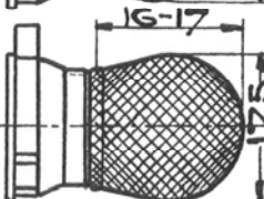
GLÖDNÄT GNAB-15 FÖR 15-LIT. BRÄNNARE
