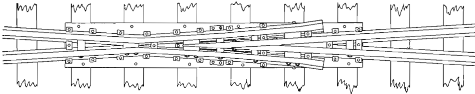
d) Dubbelspetsade korsningar.
