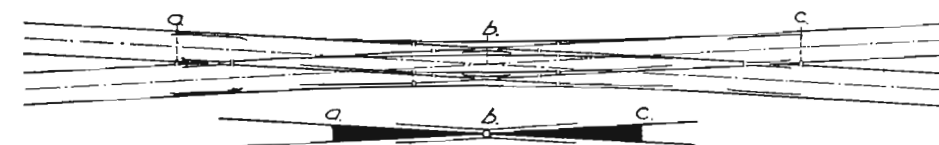
Bild 106. Dubbel korsningsväxel.
