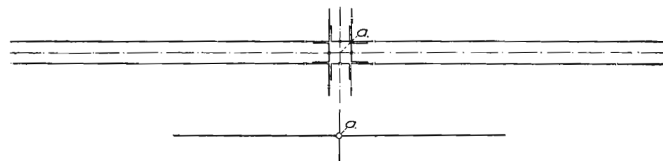
Bild 108. Spårkorsning.
