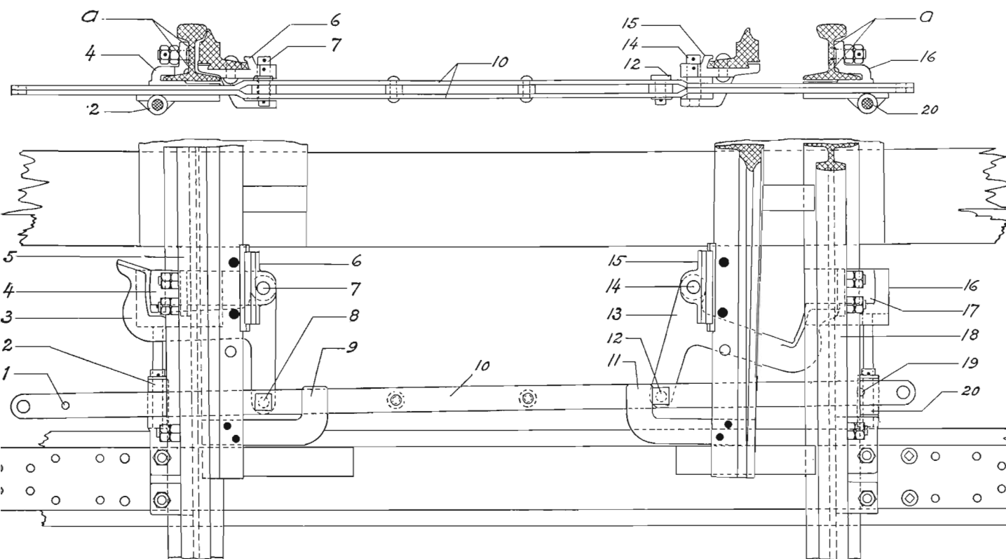
Bild 138. Hakväxellås.
