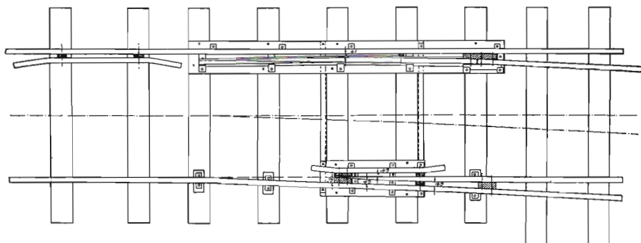
Bild 111. Entungig växel.
