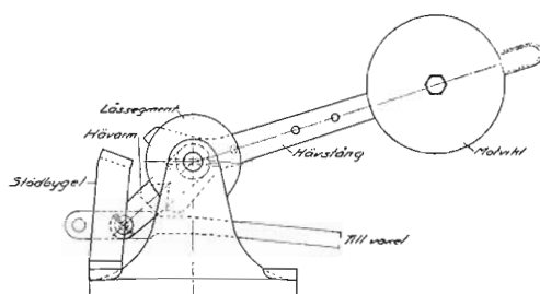
Bild 130. Växeltäll för växel utan växellås.
