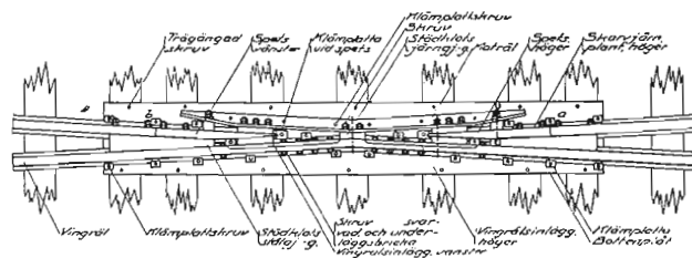
Bild 125. Dubbelspetsad korsning med spetsar och vingrälsinlägg av manganstål.
