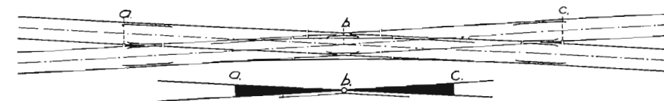
Bild 105. Enkel korsningsväxel.
