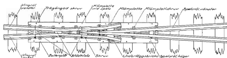
Bild 120. Enkelspetsad korsning av räl.
