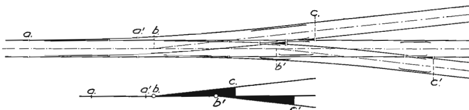
Bild 102. Tvåsidig osymmetrisk växel.
