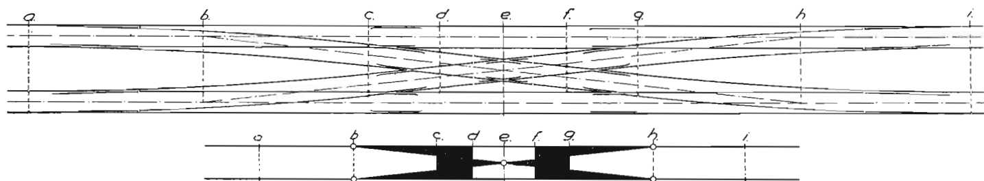
Bild 109. Kryssväxel.
