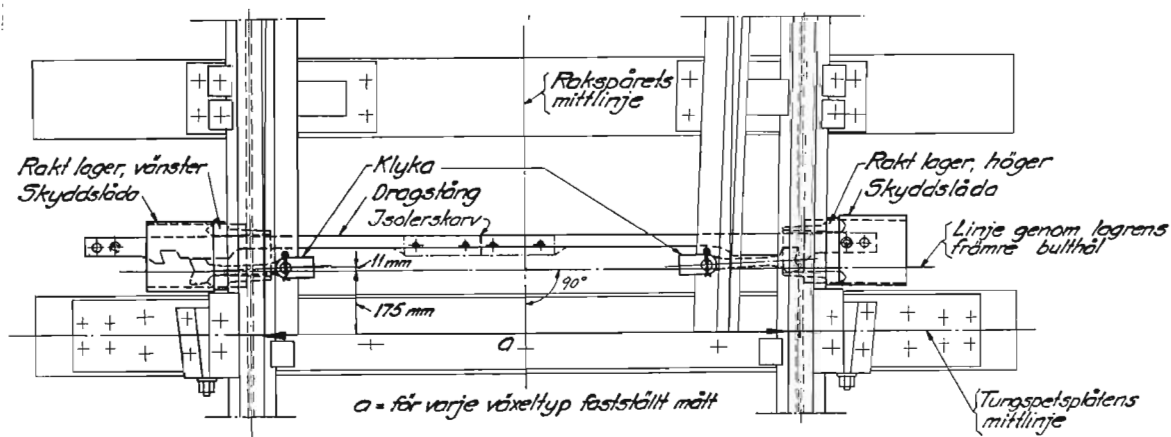
Bild 139. Klykväxellås.
