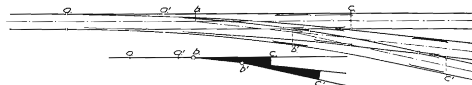
Bild 103. Ensidig tredelig växel.
