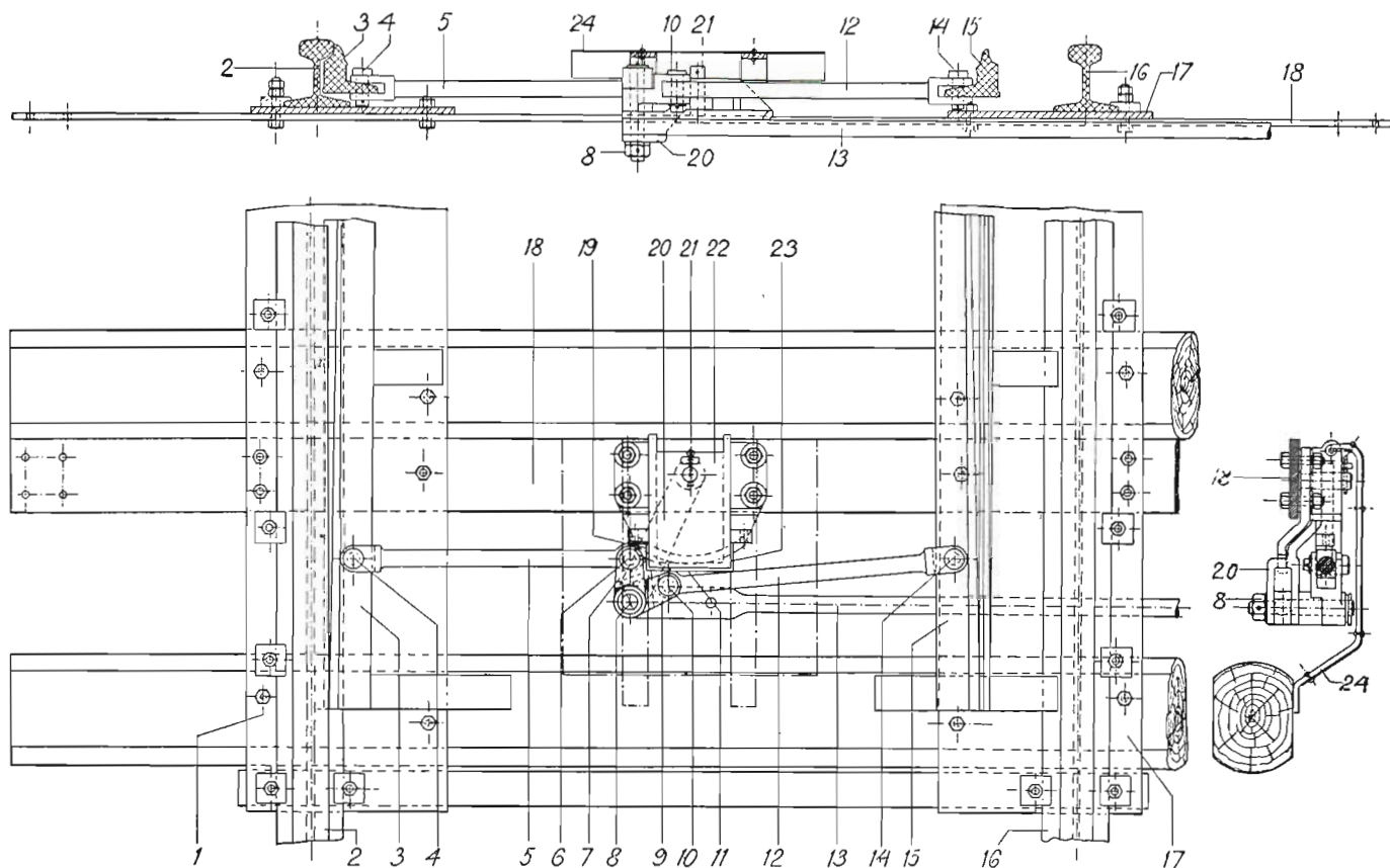
Bild 137. Länkväxellås.
