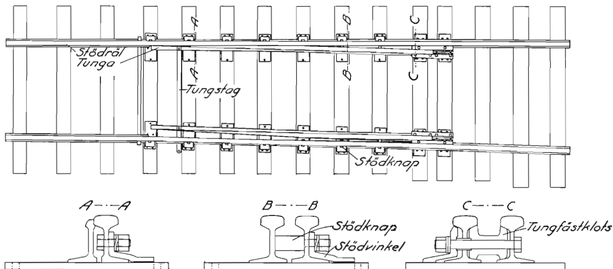
Bild 112. Tunganordning, äldre modell.
